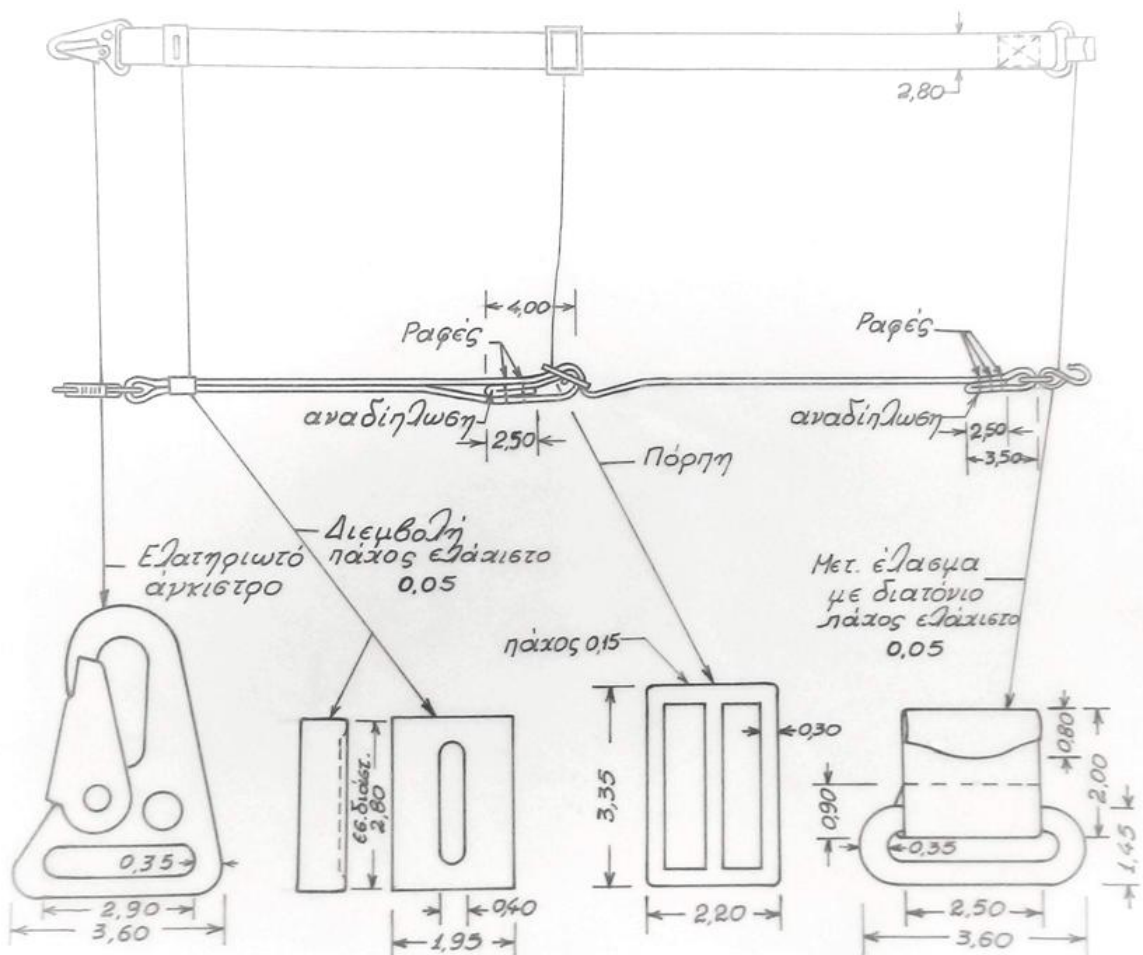
Σχέδιο 1: Κατασκευαστικά σχέδια αορτήρα τυφεκίων G3A3-G3A4
